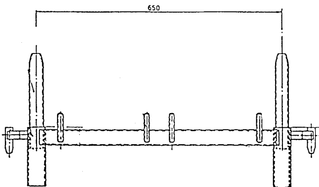
Hängetraverse für RUX-SUPER 65
