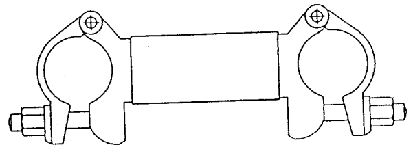
Achsmaß 180 mm
